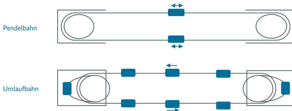
Abbildung 10: Funktionsprinzip Seilschwebbahnen
